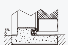
密封底邊框
