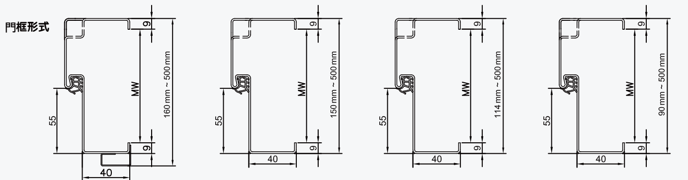
防火門 HCA 90
