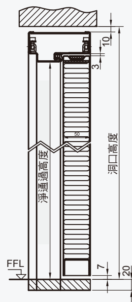
多用途門縱向視圖
