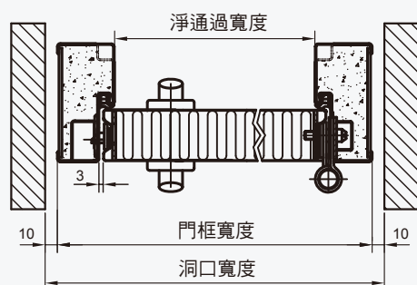
單開多用途縱向視圖
