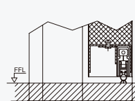
可沉降式底部密封
