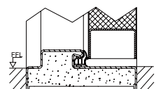
密封底邊框
