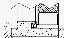
密封底邊框
