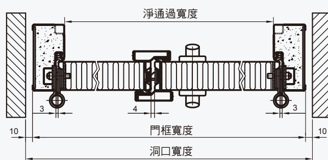
雙開多用途縱向視圖
