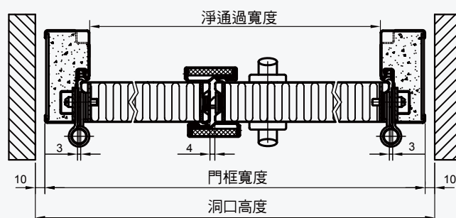
雙開防火門橫向視圖
