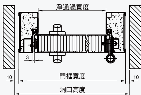
單開防火門橫向視圖
