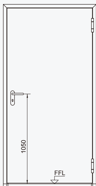
單開門視圖
