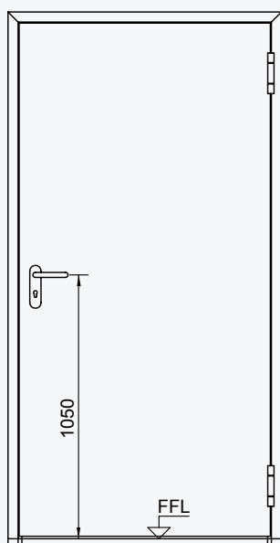
單開門視圖
