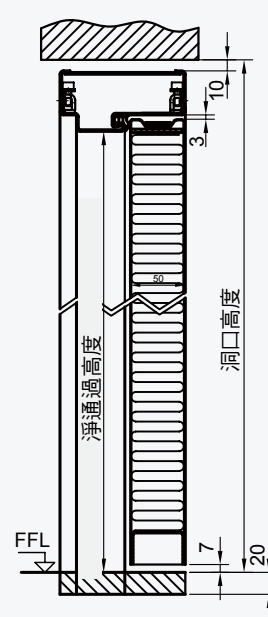
防火門縱向視圖
