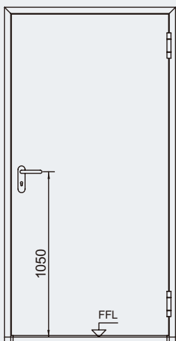
單開門視圖
