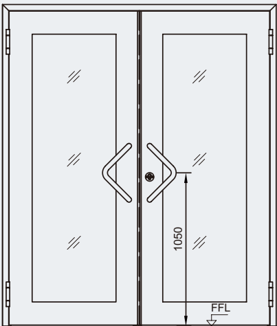
雙開門視圖
