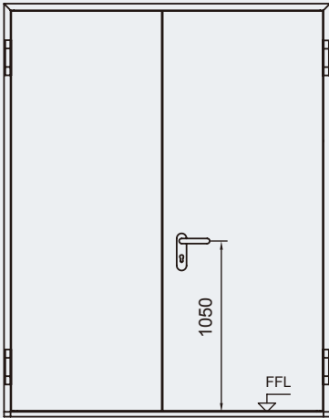
雙開門視圖
