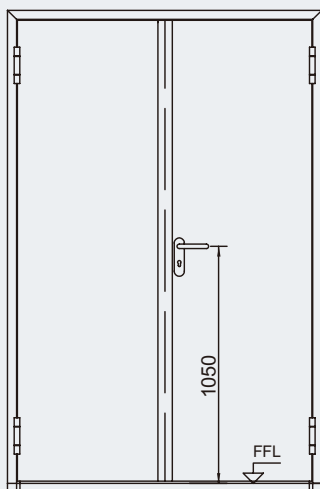
雙開門視圖
