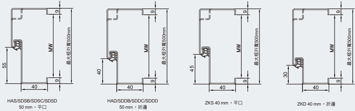
門框形式
