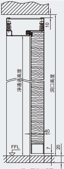
ZKS 平口門縱向視圖
