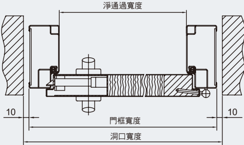
ZKD-1 折邊單開門橫向視圖
