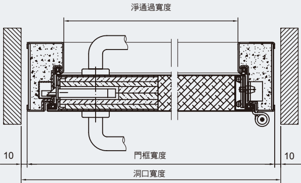
HC60SDC-1 單開門橫向視圖
