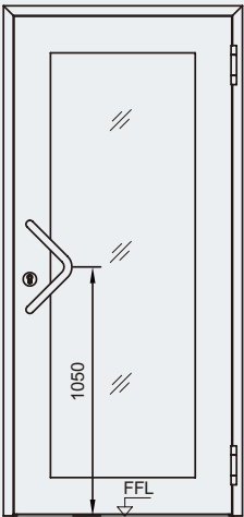
單開門視圖
