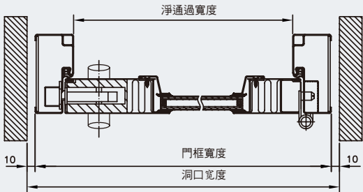
橫向視圖：HE-1
