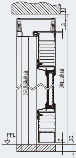
縱向視圖
