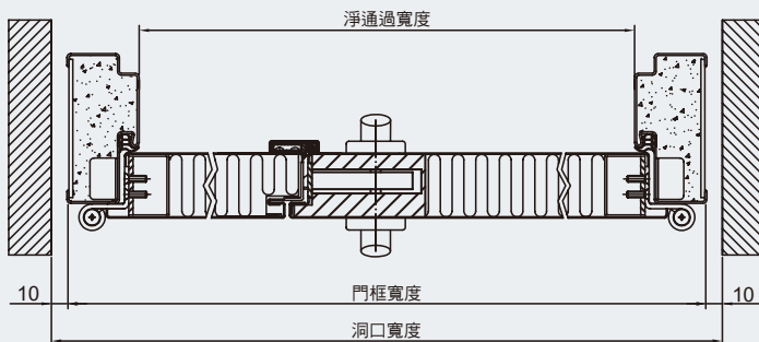
HAD-2 折邊雙開門橫向視圖
