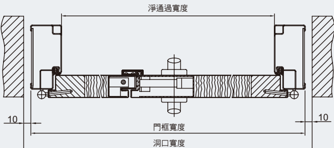
ZKD-1 折邊雙開門橫向視圖
