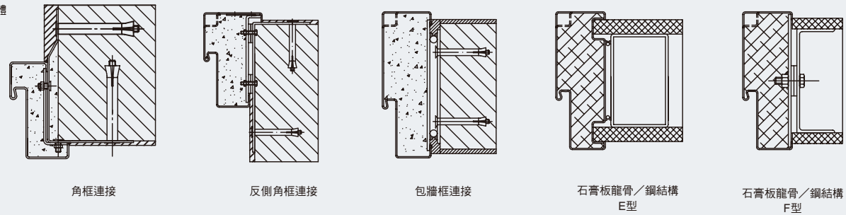
特殊安裝方式 混凝土／磚牆／特殊牆體
