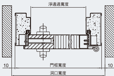
HAD-1 折邊單開門橫向視圖
