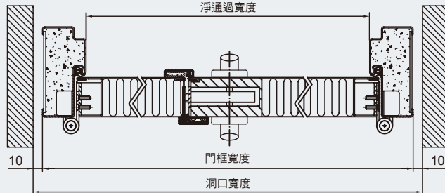
HAS-2 平口雙開門橫向視圖
