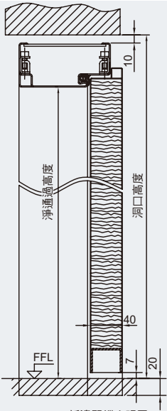
ZKD 折邊門縱向視圖
