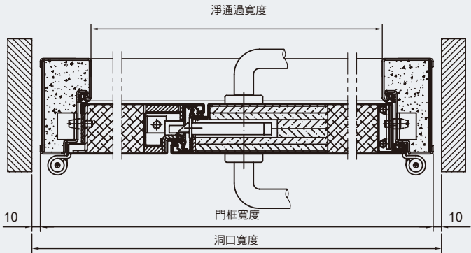
HC60SDC-2 雙開門橫向視圖
