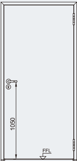
單開門視圖
