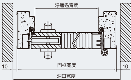
HAS-1 平口單開門橫向視圖
