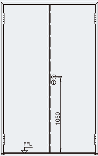
雙開門視圖
