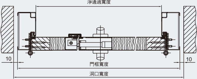
ZKS-2 平口雙開門縱向視圖
