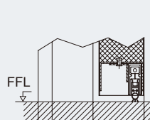
可沉降式底部密封
