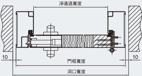
ZKS-1 平口單開門橫向視圖
